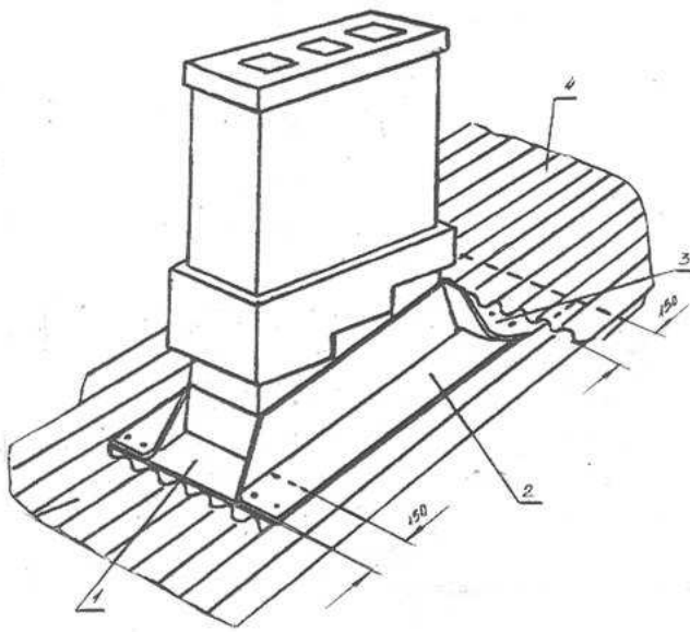
Рисунок 3 - Устройство воротника оголовка трубы
