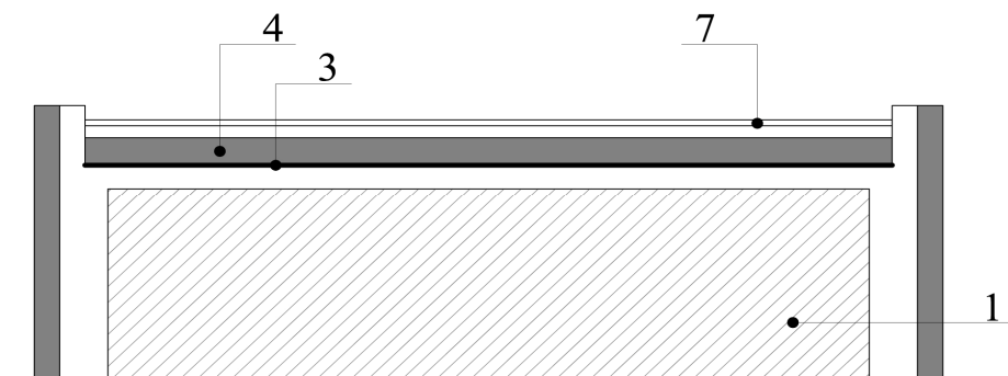
г - утепленная совмещенная плоская крыша
