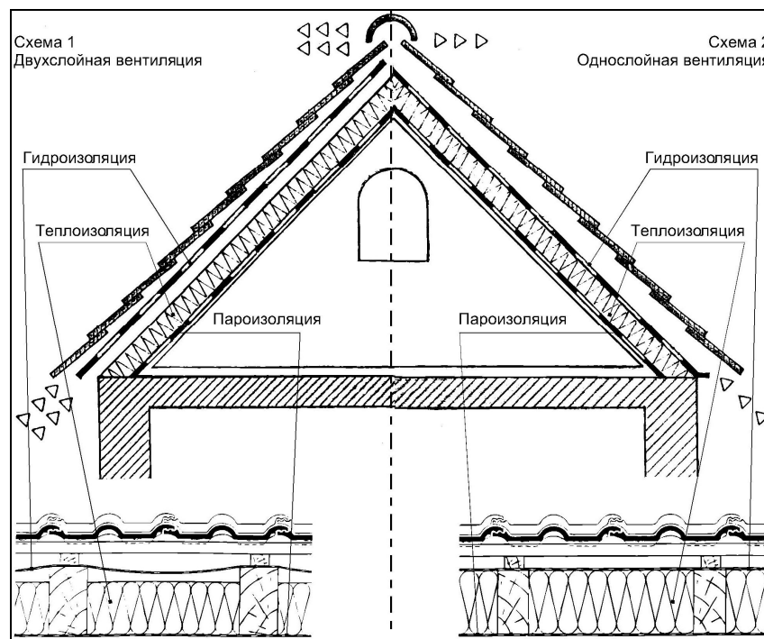
Рисунок К.1. Типы вентиляции подкровельного пространства
