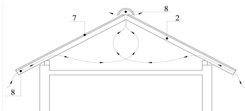
д - холодная скатная крыша
