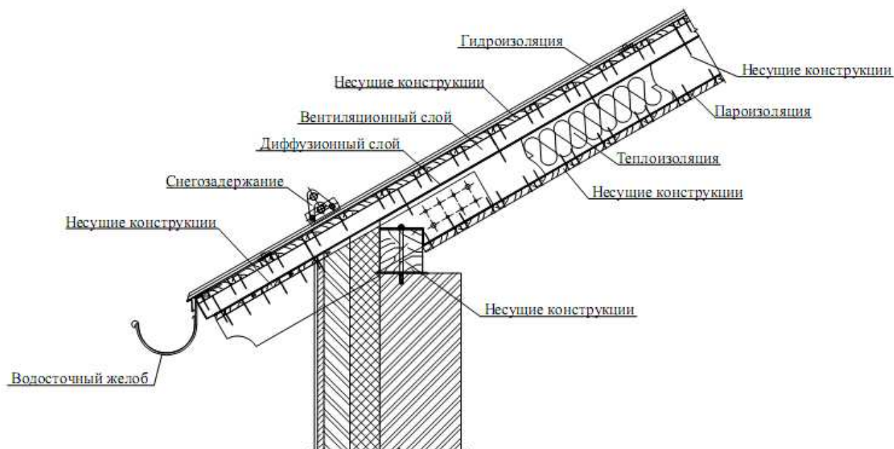
Рисунок 1. Слои скатной крыши.
