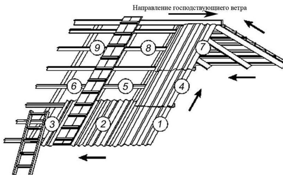
Рисунок 1 - Схема укладки хризотилцементных листов по двухпролетной схеме
