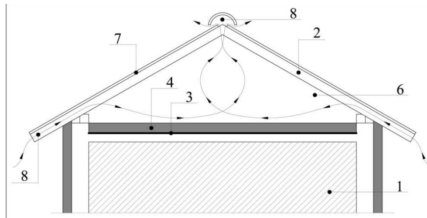
а -- утепленная чердачная скатная крыша (с холодным чердаком)
