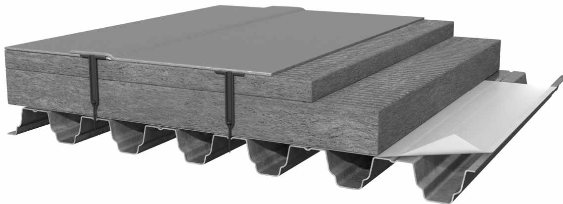
Рисунок 5 - Механическое крепление мембраны, уложенной на утеплитель.
