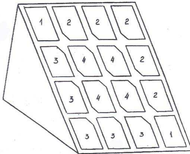
Рисунок 2 - Схема раскладки волнистых хризотилцементных листов с обрезанными углами справа налево
