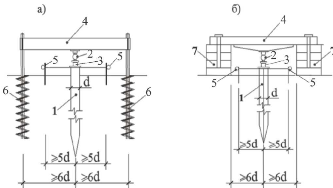
Рис. 59. Схемы установок для испытания натуральных НПСн статической вдавливающей нагрузкой: 1- НПСн; 2- образцовый динамометр; 3- гидравлический домкрат; 4- упорная балка; 5- прогибомер; 6- винтовые анкеры; 7- пригрузы платформы.
