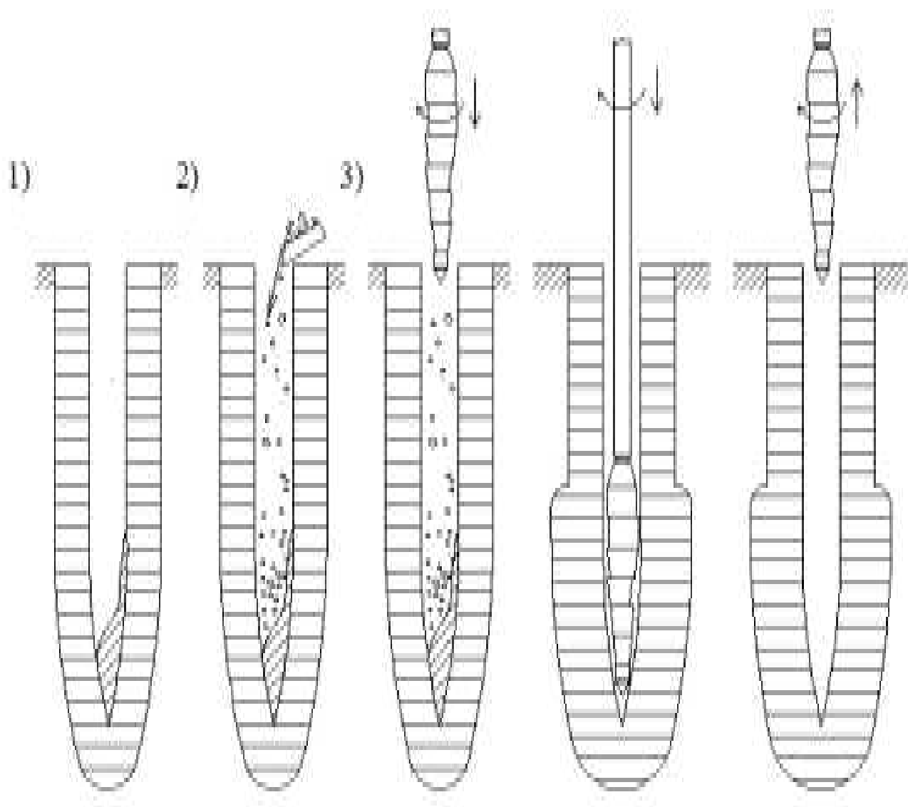
Рис. 25. Схема восстановления ствола раскатанной скважины при локальной потере устойчивости.
