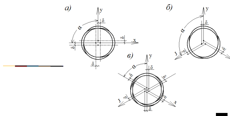
Рис. 31. Конструктивная схема РСу: 1- хвостовик; 2- формирующие сегменты; 3- раскатывающие сегменты; 4- наконечник; 5- острие; \delta - смещение сегментов относительно продольной оси ( z ); \alpha - угол разворота сегментов относительно друг друга; x, y, j - оси поперечного сечения.
