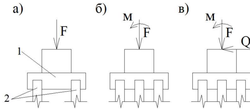
Рис. 54. Схемы передаваемых на системы «НПСн – фундамент» нагрузок: 1- фундамент; 2- НПСн.
