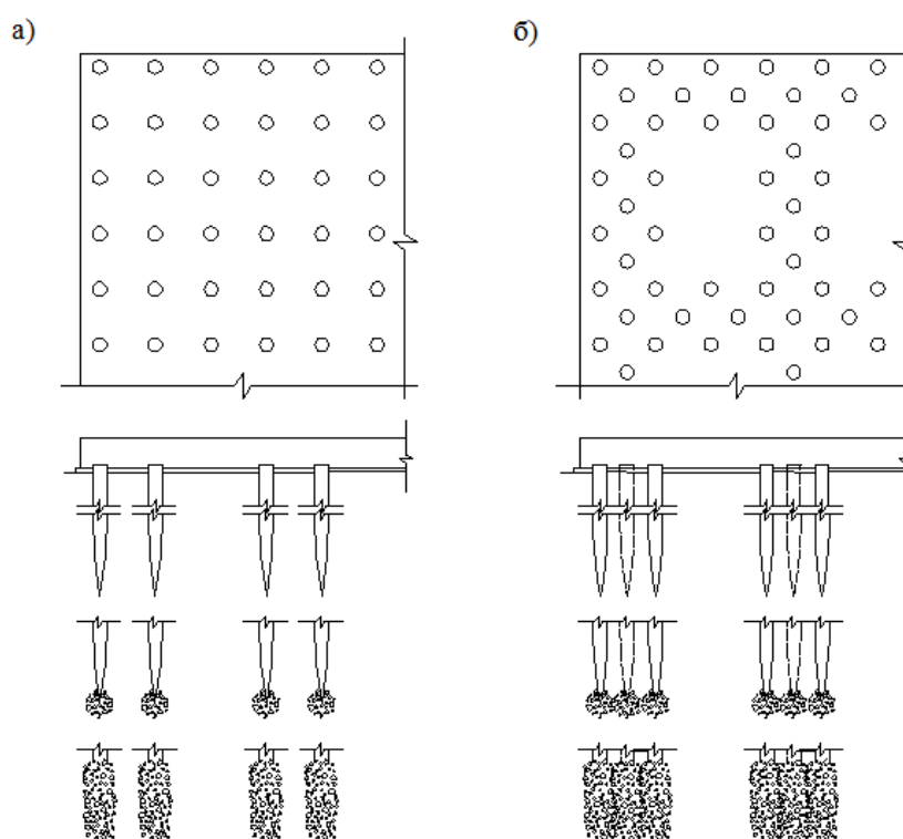
Рис. 57. Конструктивные схемы монолитных плитных фундаментов на основаниях из НРСн сплошных свайных полей (а) и прерывистых (б).
