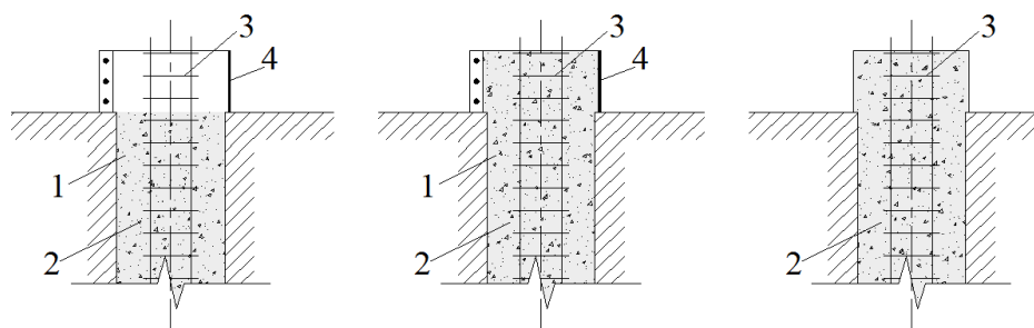
Рис. 46. Технологическая схема устройства оголовка НРСн в инвентарной опалубке: 1- раскатанная скважина; 2- свежееуложенная бетонная смесь; 3- арматурный каркас; 4- опалубка.
