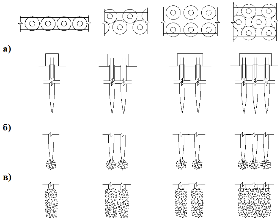
Рис. 55. Конструктивные схемы монолитных ленточных фундаментов из НПСн: а) НПСо; б) НПСу; в) НПСк.
