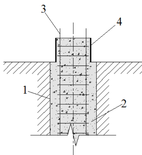
Рис. 47. Конструктивная схема устройства оголовка НРСн в несъемной опалубке: 1- раскатанная скважина; 2- свежеуложенная бетонная смесь; 3- арматурный каркас; 4- опалубка.
