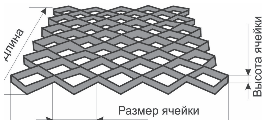
б) схема растяжения объемной георешетки
